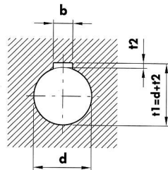
DIN 6885/2
