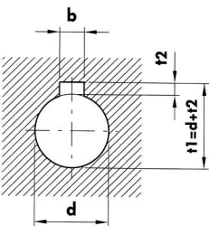
DIN 6885/1
